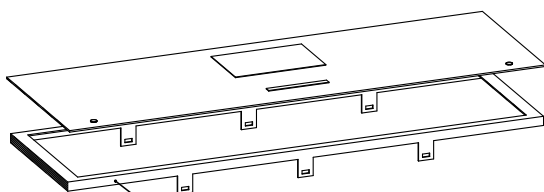
Sicherheitsabdeckung aus Aluminium mit zwei Schließern (als Innenabdeckung verwendbar, auch für nachträglichen Einbau geeignet)
