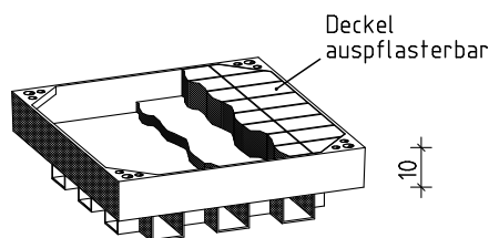
Einführungsrahmen 91/25/9 cm
