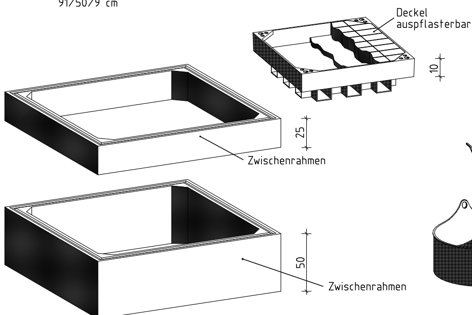
Einführungsselement 91/50/9 cm
